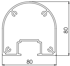
Mono-D (D-Profile) 90
