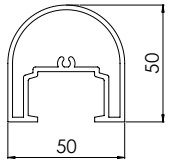
Mini-D (D-Profile) 90
